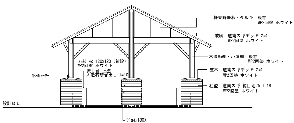
東西側立面図 A1:1/50 A3:1/100
