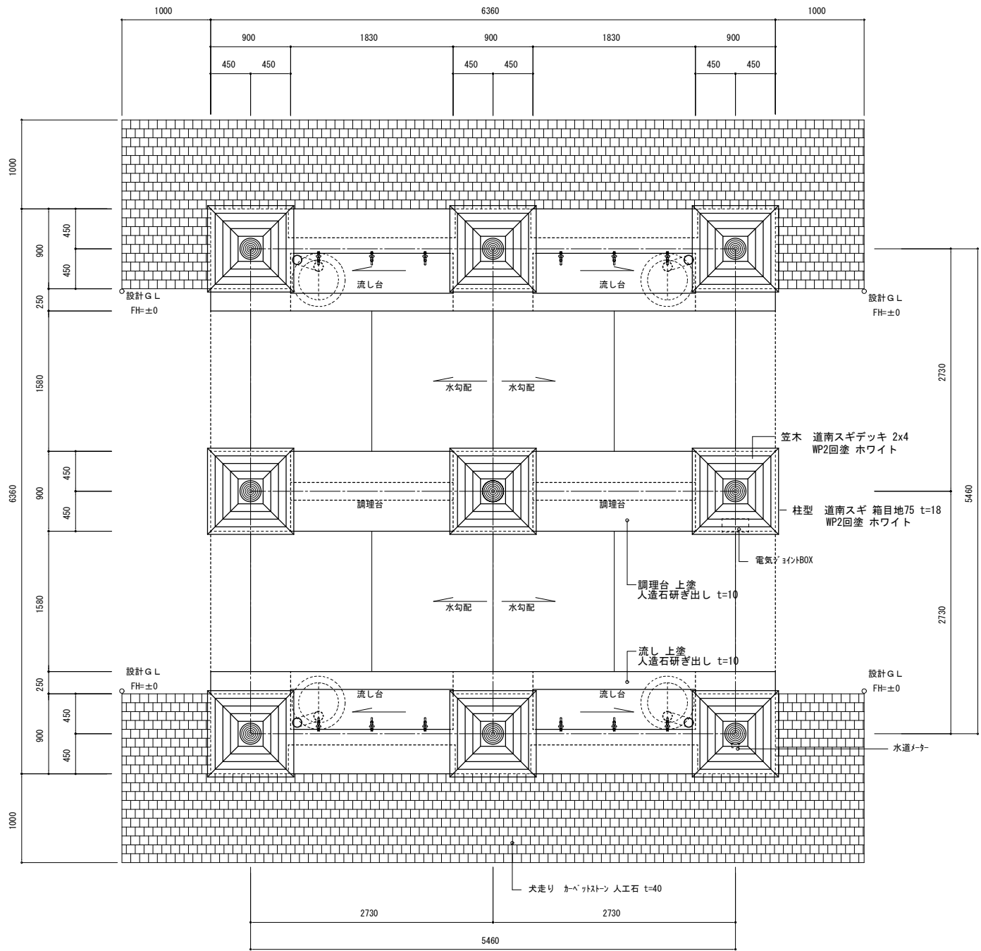
炊事棟平面図 A1:1/30 A3:1/60
