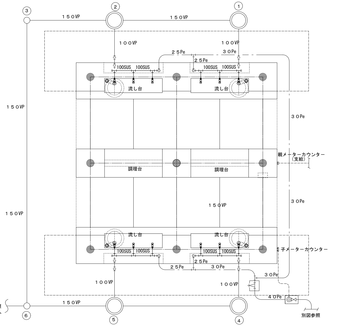
炊事棟 2 給排水設備平面図 A1:1/30 A3:1/60
