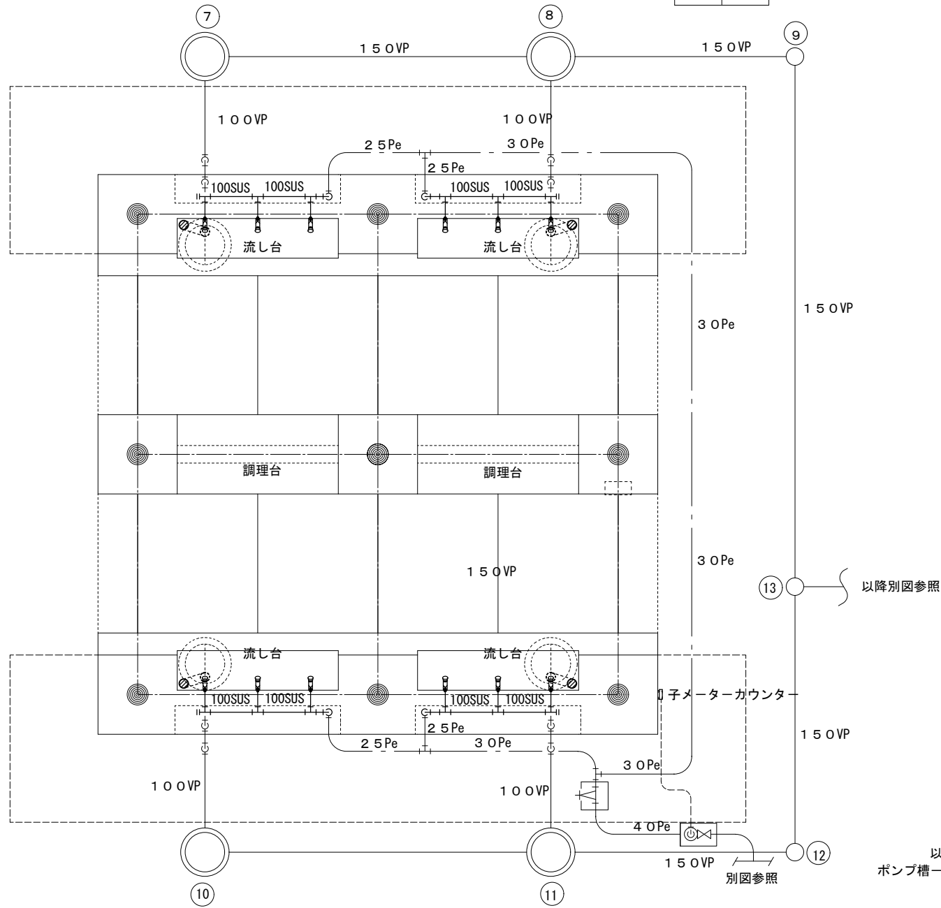
炊事棟 1 給排水設備平面図 A1:1/30 A3:1/60
