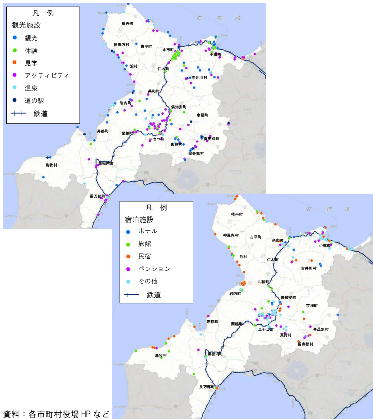
図 3-22 後志地域の観光・宿泊施設
