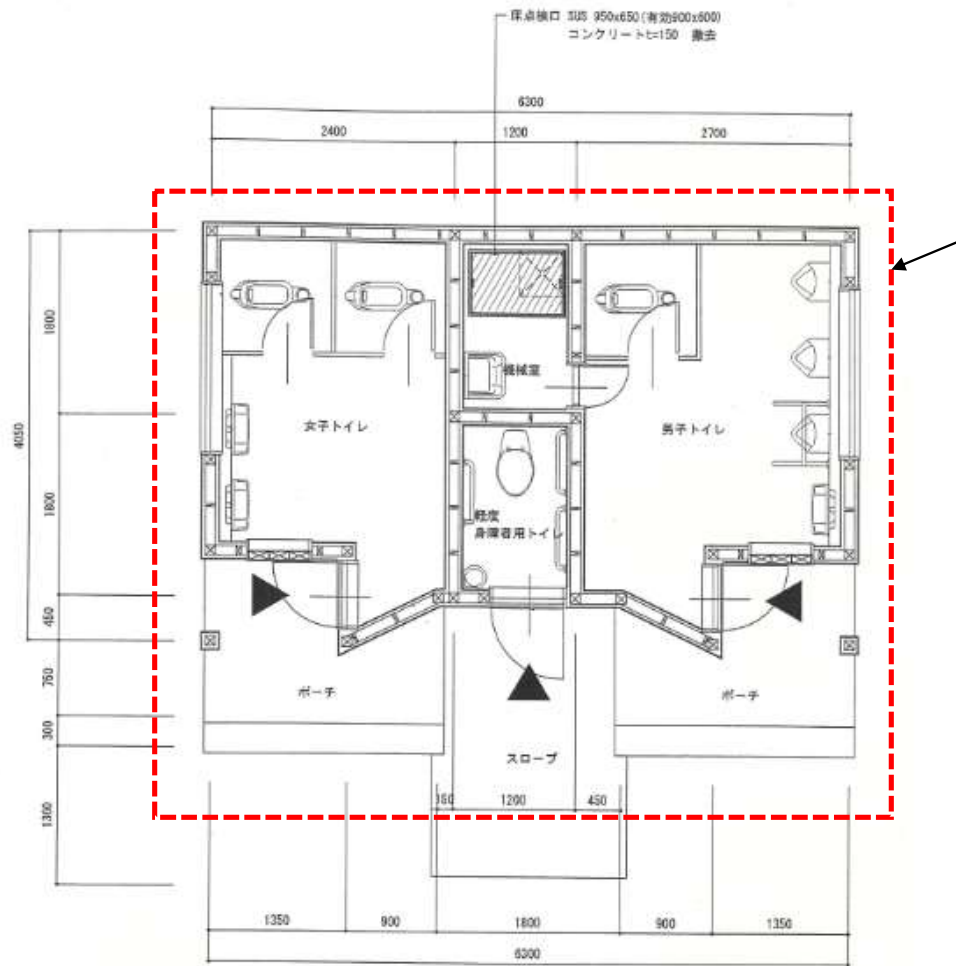
既設トイレ平面図 S-1/50
